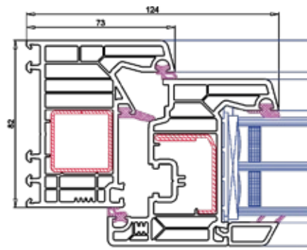
Sección lateral
